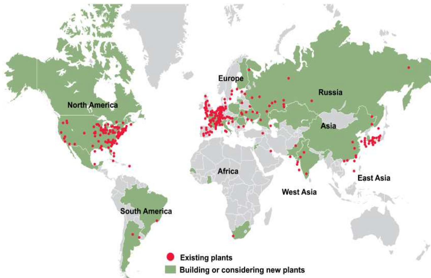
Harta răsparidii centralelor nuclearo-electrice în lume și a viitoarelor amplasamente.
