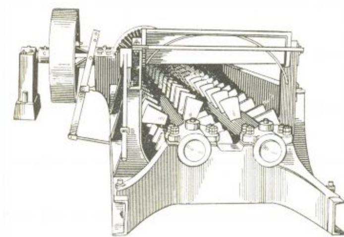
Amestecător cu două valțuri.
