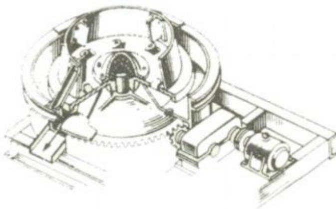
Strung pentru așchieria argilei.
