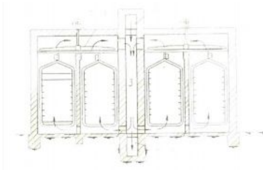
Uscător tip tunel cu recircularea agentului termic.
