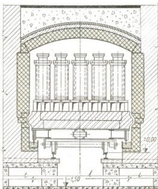
Cuptor tunel pentru arderea conductelor.
