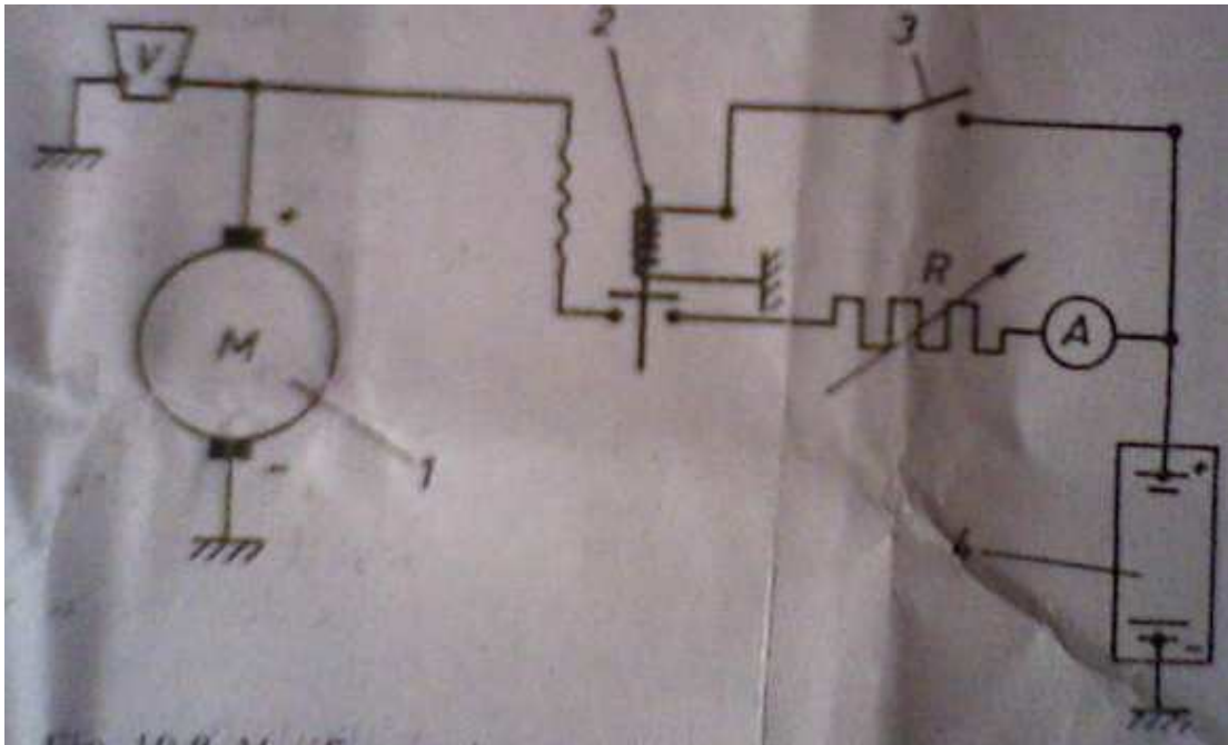
Fig 10.8. Verificarea demarorului pe stand (schema de montaj)
