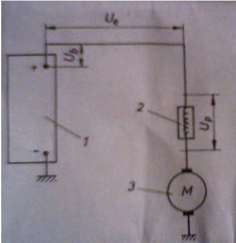
Fig 10.7. Schema verificării caderilor de tensiune în circuitul de pornire cu demaror
